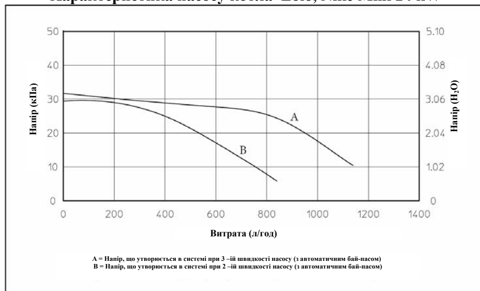
Характеристика насоса котла Eolo, Nike Mini 24 kW
