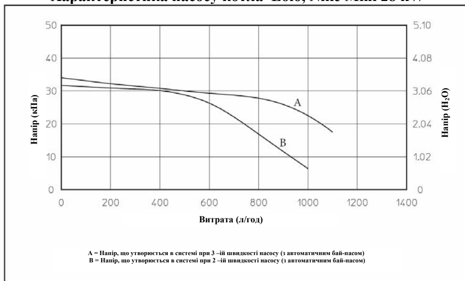
Характеристика насоса котла Eolo, Nike Mini 28 kW
