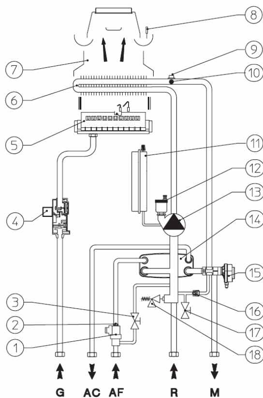
Гідравлічна схема котла Nike Mini 24 kW – 28 kW
