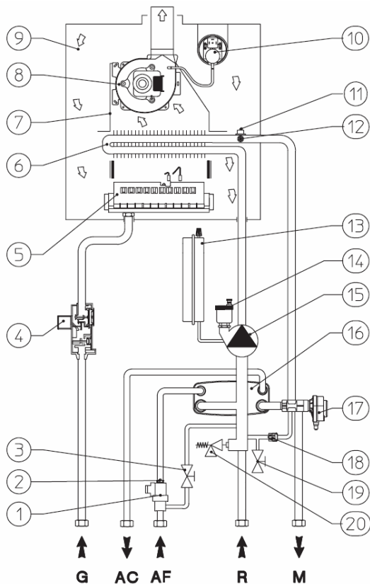
Гідравлічна схема котла Eolo Mini 24 kW – 28 kW
