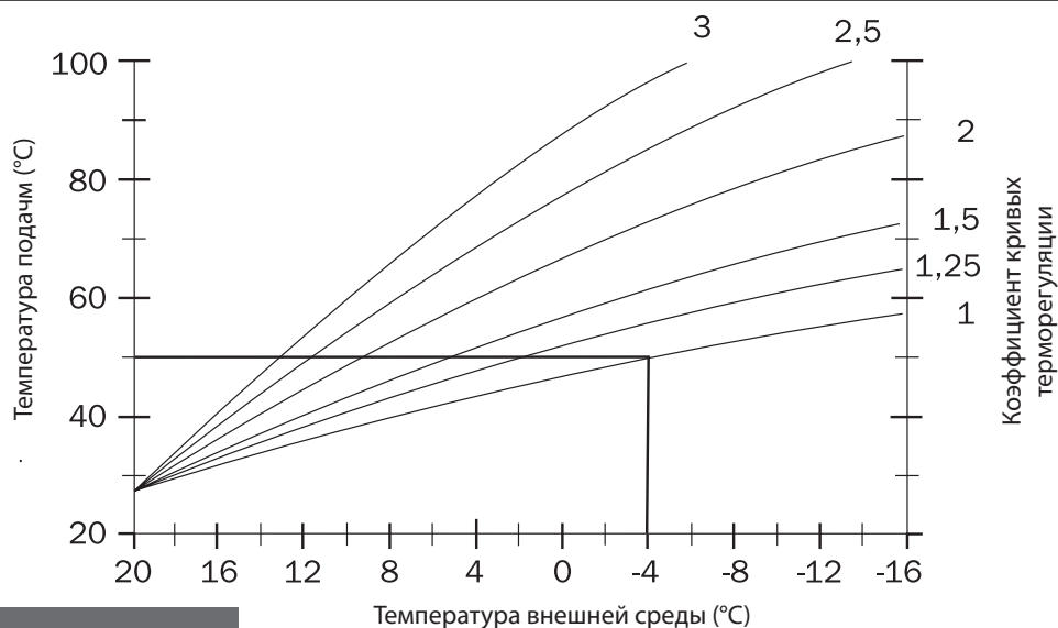
рис. 2 - Кривые терморегуляции
