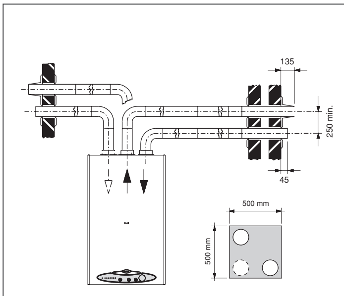
рис. 20 - Примеры установки с отдельными трубами
