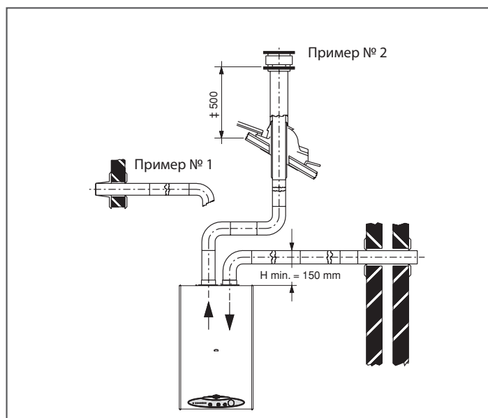
рис. 19 - Примеры установки с отдельными трубами
