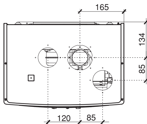
Вид сверху
