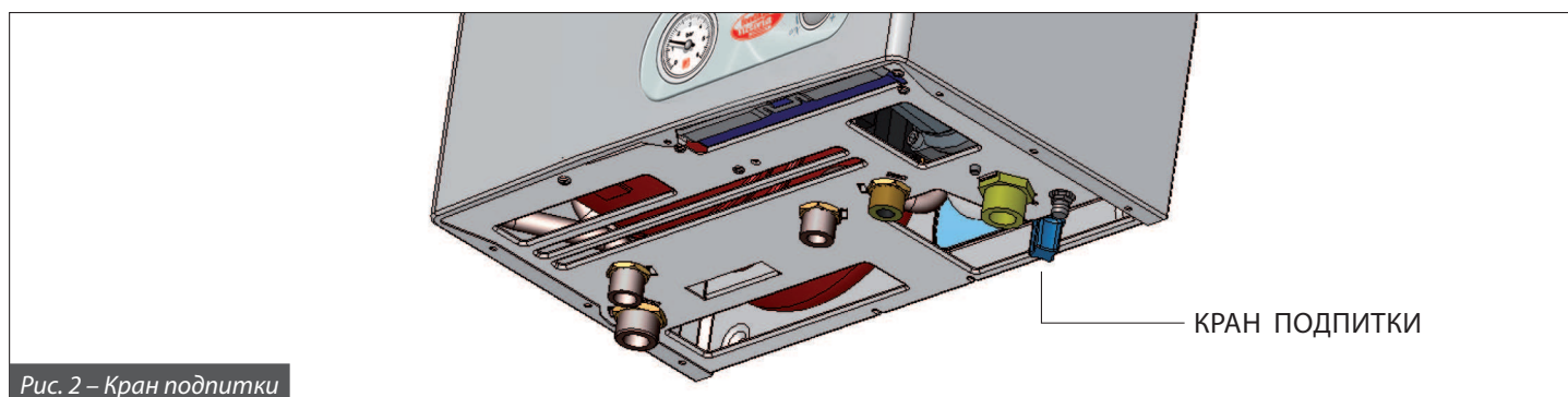
Рис. 2 – Кран подпитки
