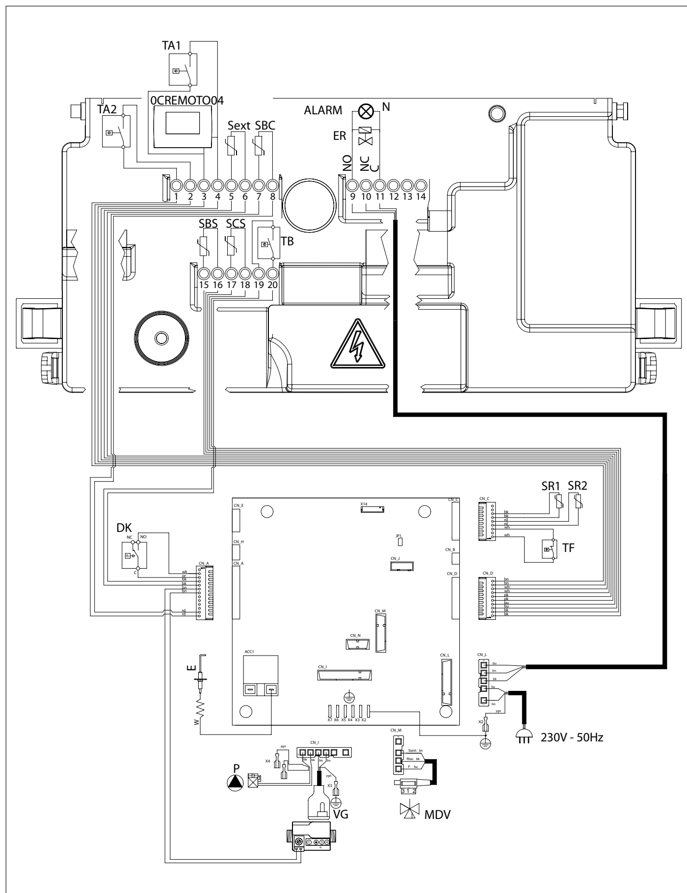
Рис. 29 Электрическая схема RBTN
