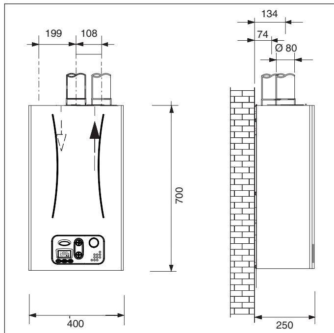
Рис. 17 Размеры для подсоединения раздельных труб воздухоподачи/дымоотвода
