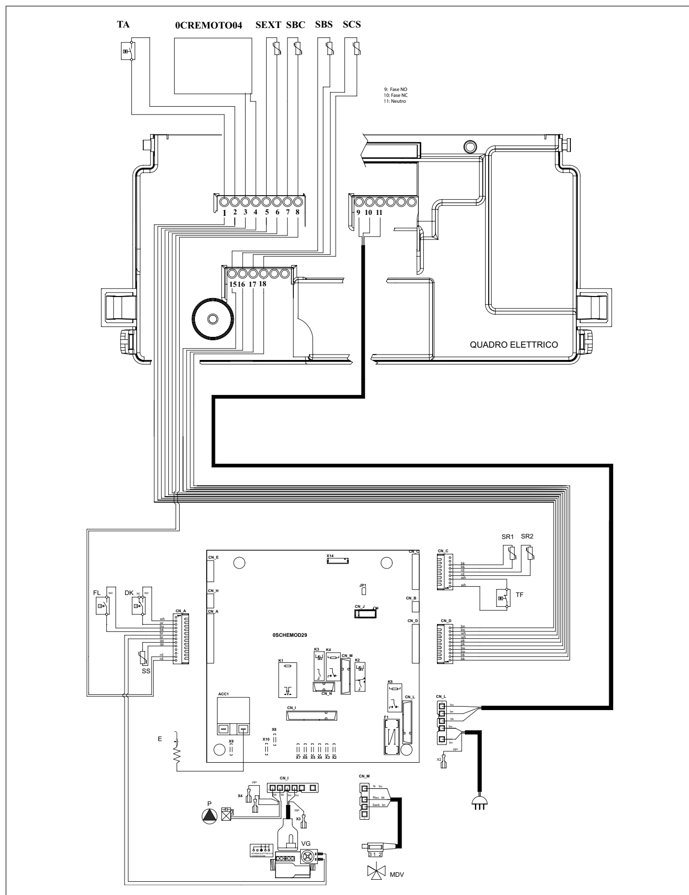
Рис. 27 Электрическая схема CTN
