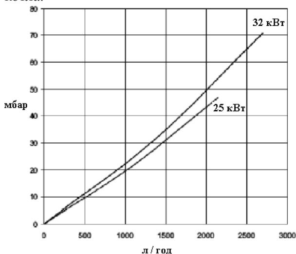
Втрата напору в котлі
