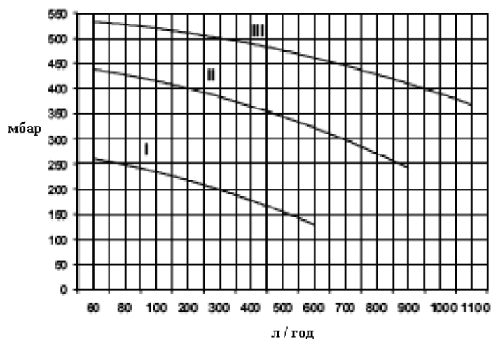
Характеристики циркуляційного насоса
