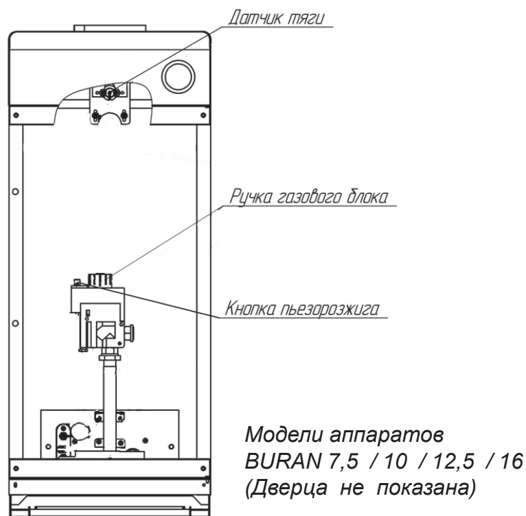
Рисунок 2 - Особенности котлов BURAN с газовым блоком 630 EUROSIT
