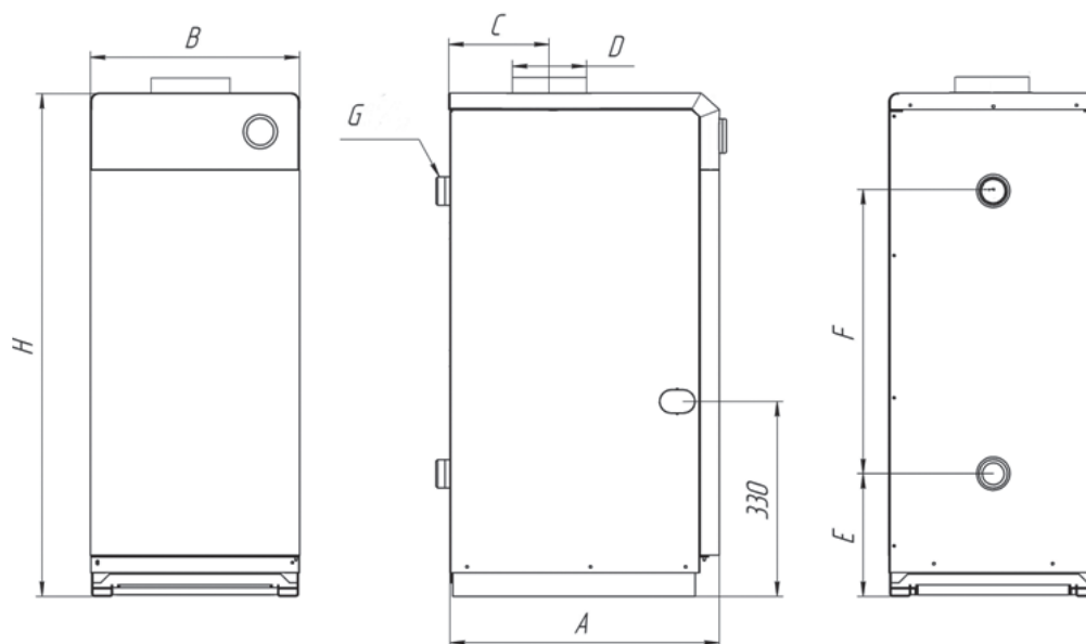
Рисунок 1 - Общий вид, габаритные и присоединительные размеры котлов BURAN 7,5/ 10/ 12,5/ 16/ 20/ 25/ 30
