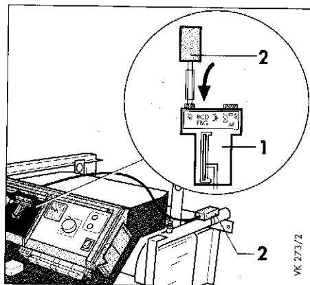
Рис. 6.8 Подключите датчик подающей линии
