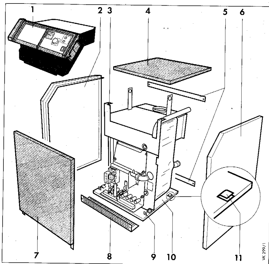
Рис. 9.2 Монтаж облицовки котла
