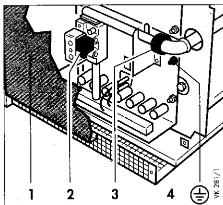
Рис. 10.4 Демонтаж горелки
