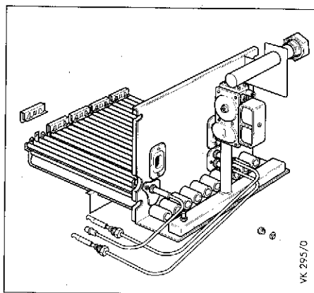
Рис. 10.2 Визуальный контроль горелки
