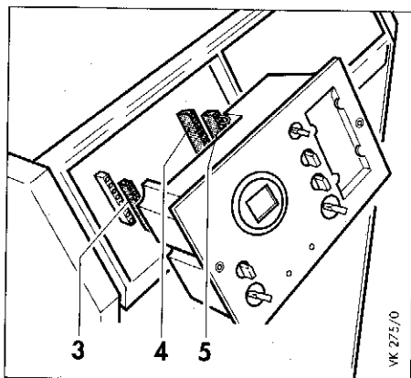
Рис. 6.9 Вставьте регулятор VRC... в панель управления котла
