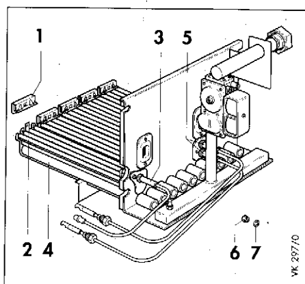
Рис. 10.5 Очистка горелки
