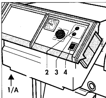
Рис. 10.1 Предохранитель котла от перегрева (STB) / Сигнальная лампа "Сбой" / Кнопка сброса состояния "Сбой" / Главный выключатель
