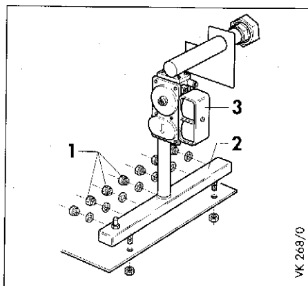
Рис. 5.8 Сопла
