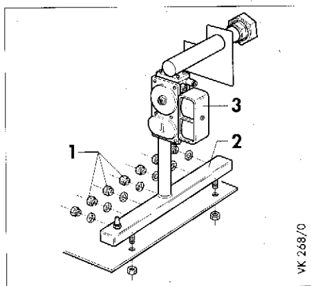
Рис. 5.7 Сопла
