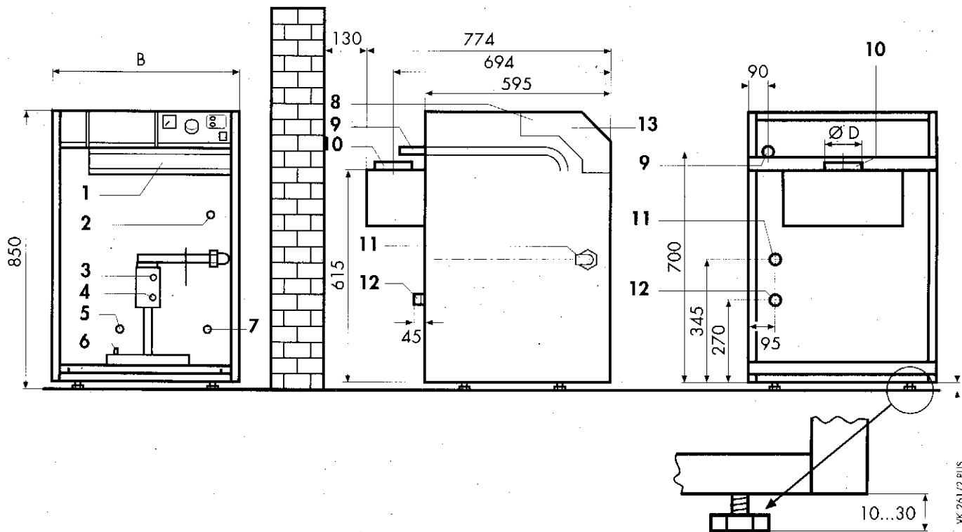
Рис. 4.1 Размеры
