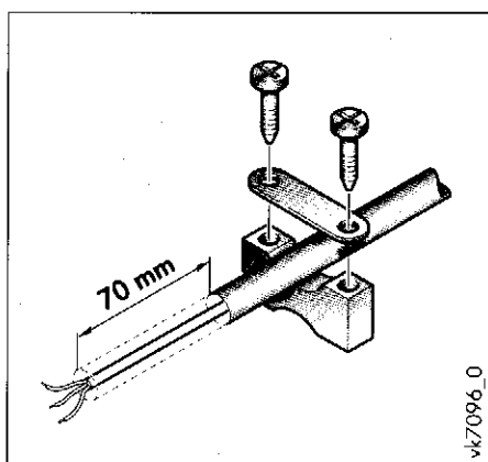
Рис. 12.2.2 Предохранители натяжения кабеля
