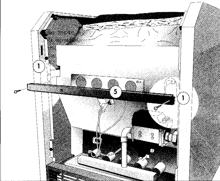
Рис. 10.2.5 Установка поперечины
