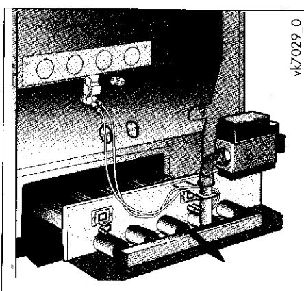
Рис. 15.2.2 Вытаскивание горелки
