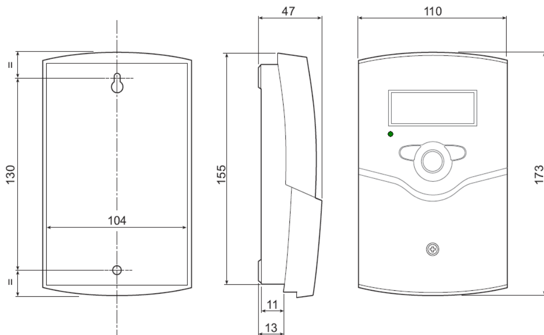
Рисунок 1 — размеры контроллера.
